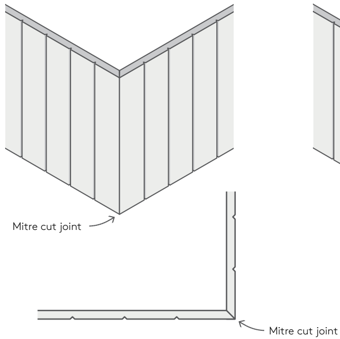
Edge Panel
